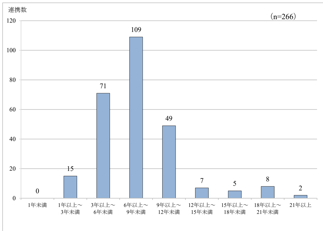
図 2.10-1 運用年数
